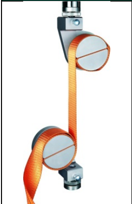
Tensile- Webbing
